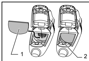
1. Esponja 2. Pared acanalada
