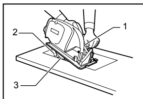
1. Palanca de retracción 2. Protector inferior 3. Disco de sierra
